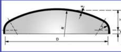
KLOPPER DIN 28011
