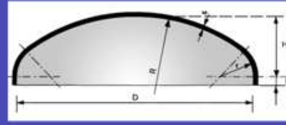
KORBBOGGEN DIN 28013
